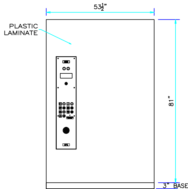
ELEVATION B
