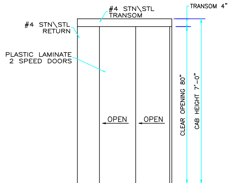
ELEVATION A
